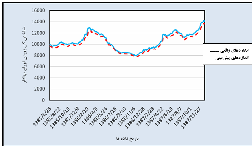
شکل شماره (۳): مقایسه بین اندازه‌های واقعی و پیش‌بینی شده الگوی (۵) ARIMA، ۱، ۰، ۵
